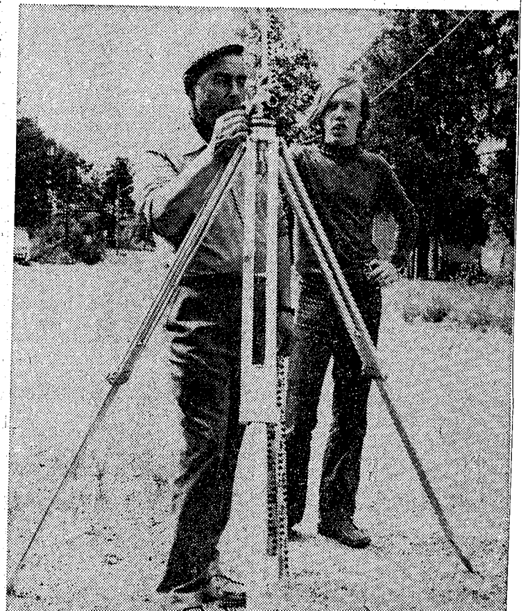
Verkmästare Edvin Danielsson och "pinnpojken" Kaj Lakså, båda från Saxdalen, i arbete med avvägning för den nya vägen.
