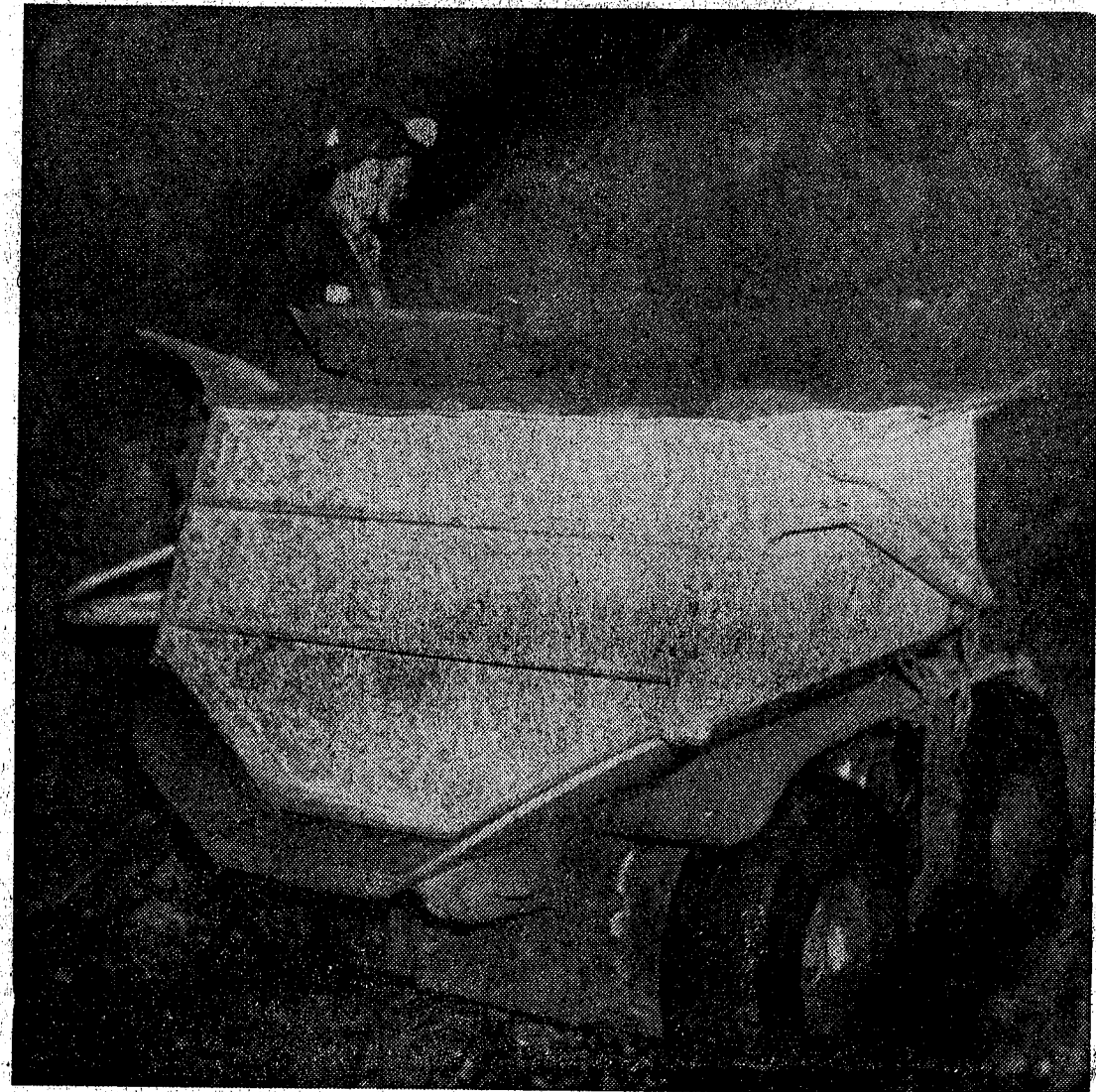
Bror Fridlund arbetar ovan med den gummihjulsförsedda last- och transportvagnen framme vid fronten.
